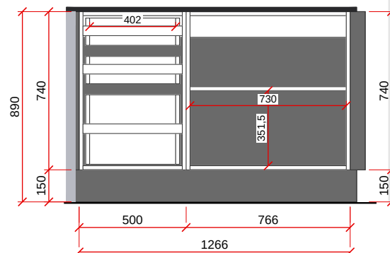
VISTA B - ESC. 1:25
